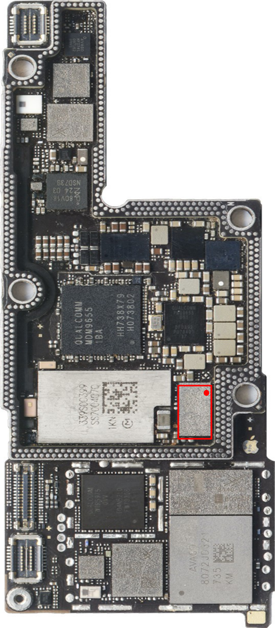
iPhoneX U_QET_E 功放供电对地阻值
